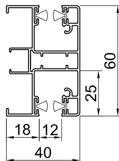
uszczelka szczotkowa
